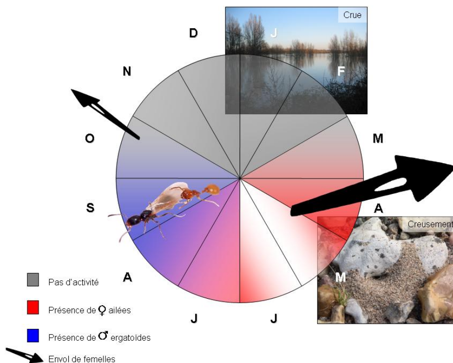
Figure 9. Cycle biologique de C. elegans (Lenoir J.-C. et Mercier J.-L., en préparation).
